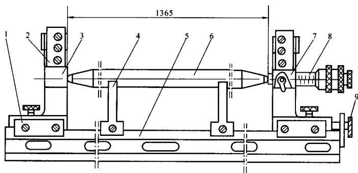
图 A.1 轮对内距尺检具结构示意图
