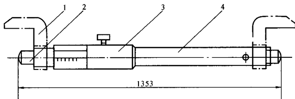
图2 标尺式轮对内距尺结构示意图
