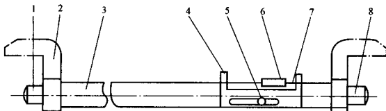
图1 数显式轮对内距尺结构示意图
